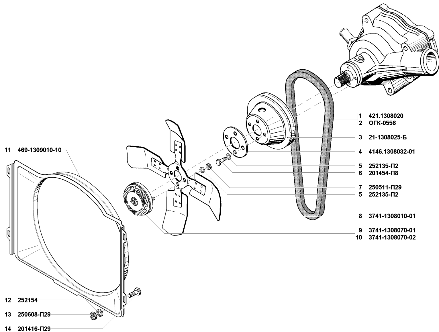
Рис. 33. Вентилятор (1308) и кожух вентилятора (1309) Fig. 33. Fan (1308) and fan housing (1309)
